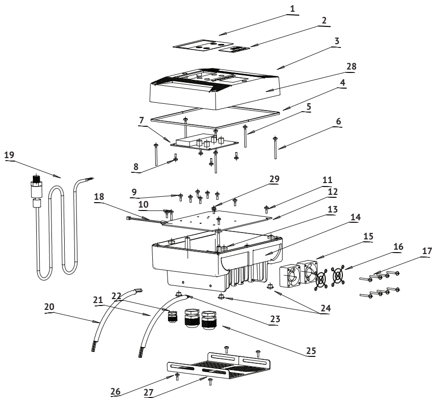
Рисунок 2 - Устройство частотного преобразователя
