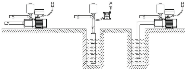
Рисунок 3 – Установка частотного преобразователя
