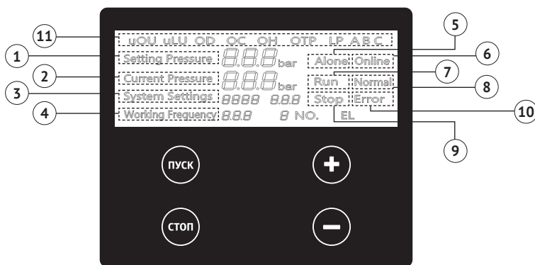
Рисунок 5 – Панель управления
