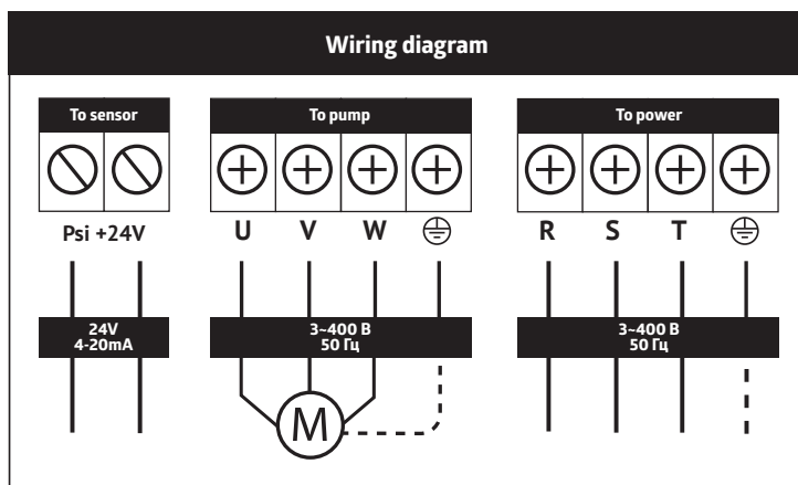
Рисунок 4 – Схема электрического подключения
