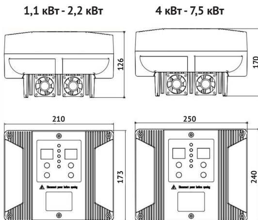
Рисунок 1 – Габаритные размеры FCP
