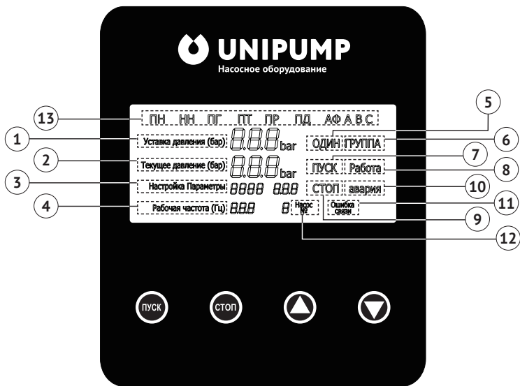
Рисунок 7 – Панель управления
