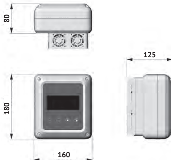
Рисунок 1 – Габаритные размеры FCP-1.1MS, FCP-1.5MS, FCP-2.2MS
