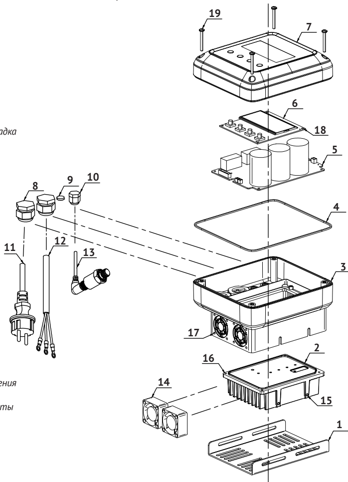
Рисунок 3 – Конструкция частотного преобразователя
