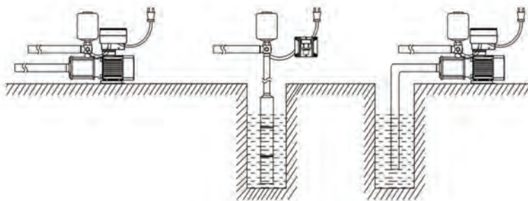
Рисунок 4 – Установка частотного преобразователя
