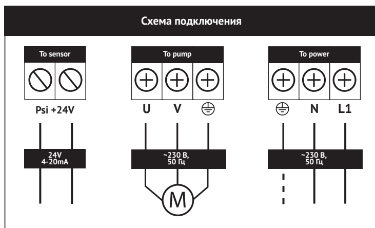
Рисунок 5 – Схема электрического подключения
