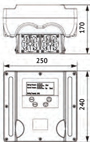
Рисунок 2 – Габаритные размеры FCP-3LM
