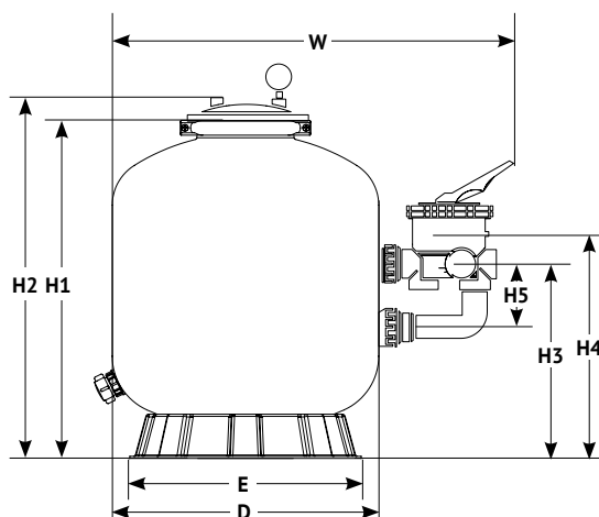
Габаритные и присоединительные размеры
