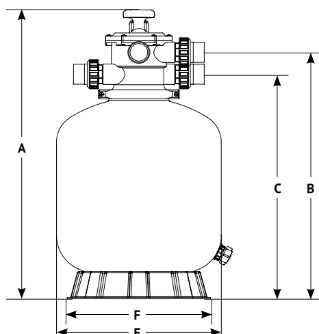
Габаритные и присоединительные размеры
