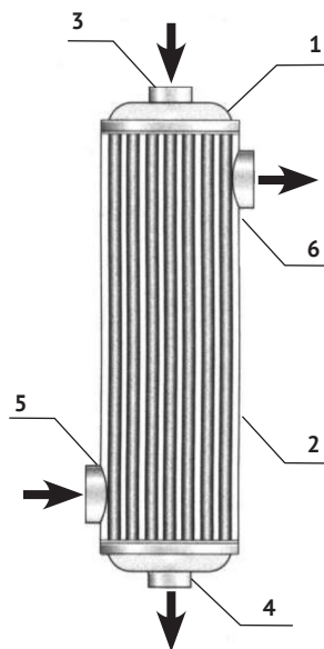
Рисунок 2 – Общее устройство теплообменника
