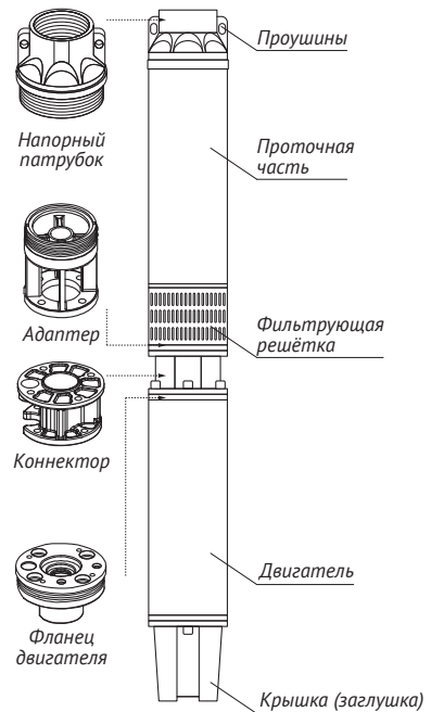
Рис. 3 - Насос 6"
