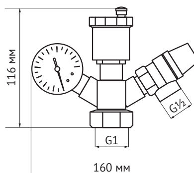
Исполнение «Слим»
