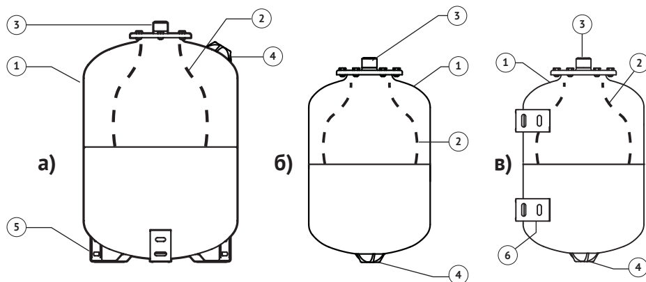
Рисунок 1 – Устройство расширительного бака
